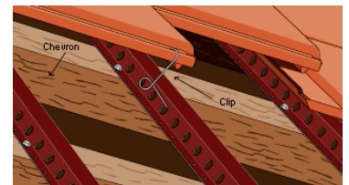
Intégration d'un pare-pluie sans contre-lattage
