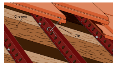
Intégration d'un pare-pluie sans contre-lattage
